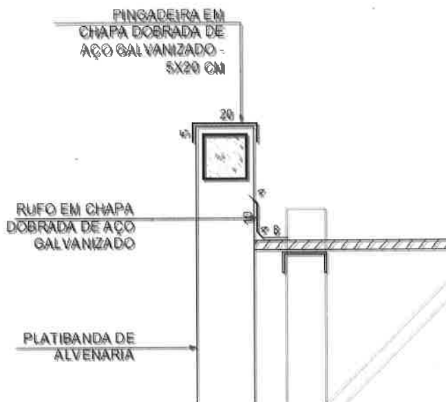
Figura 13 – imagem exemplificativa de detalhe de rufos/alvenaria e pingadeira
